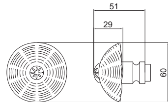
VELIKA KOVANA KUGLA ZA VRATA Br. 620000
