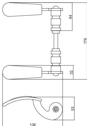
KOVANA KVAKA ZA VRATA Br. 120000
