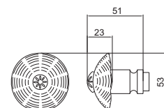
MALA KOVANA KUGLA ZA VRATA Br. 520000
