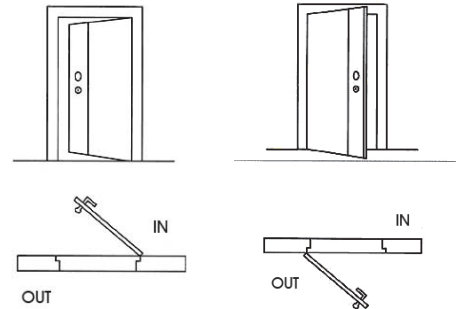
DIN Norm - LEFT OPENING
