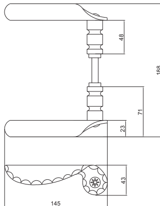
KOVANA KVAKA ZA VRATA Br. 220001
